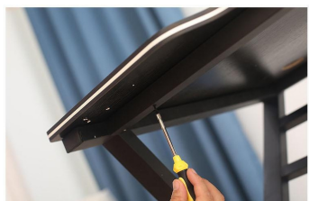
10: Uwaga - po ustaleniu pozycji naciśnij stół ręką i użyj wkrętów samogwintujących, aby dokręcić dolną część poprzeczki.
